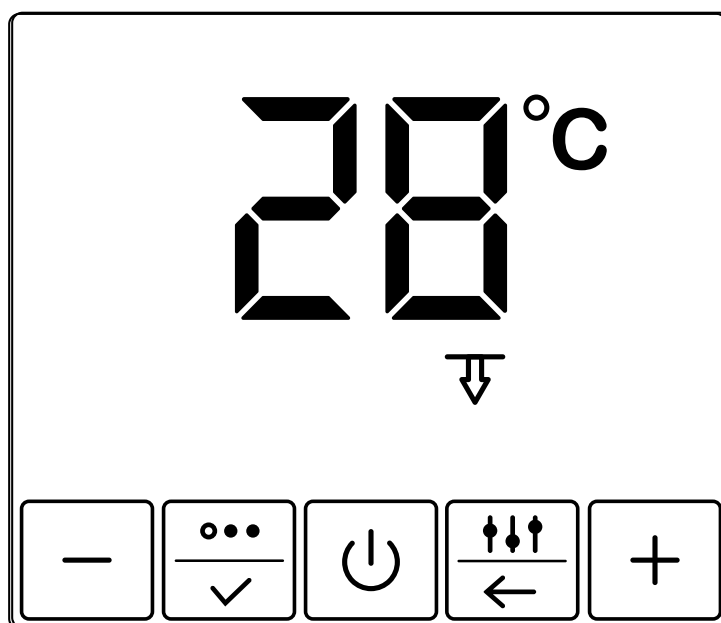
Рис. 10. Установка максимальной температуры воздуха
